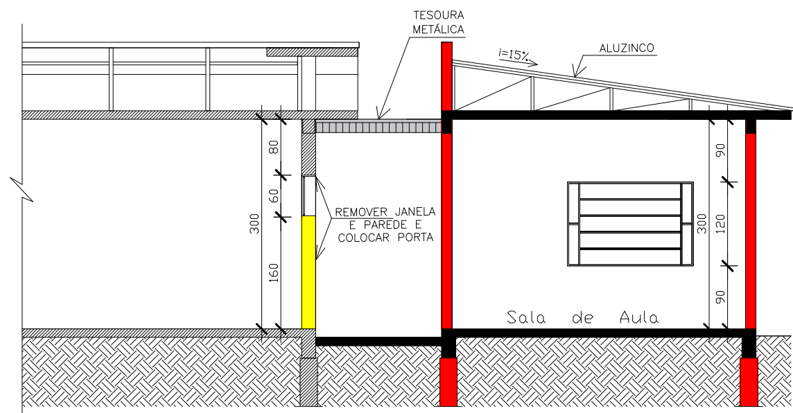
CORTE BB'
