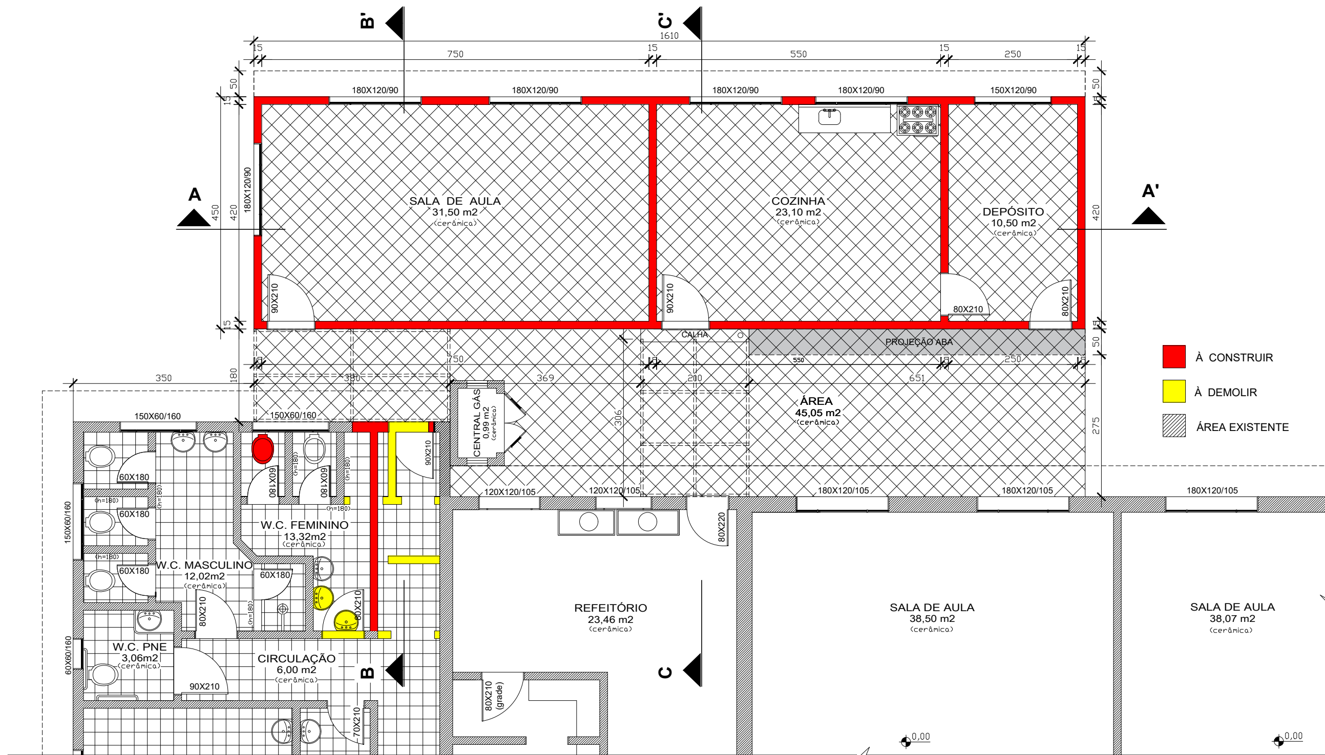
PLANTA BAIXA
