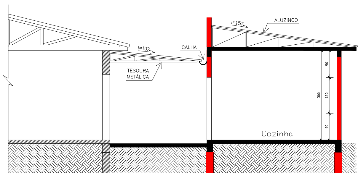
CORTE CC'
