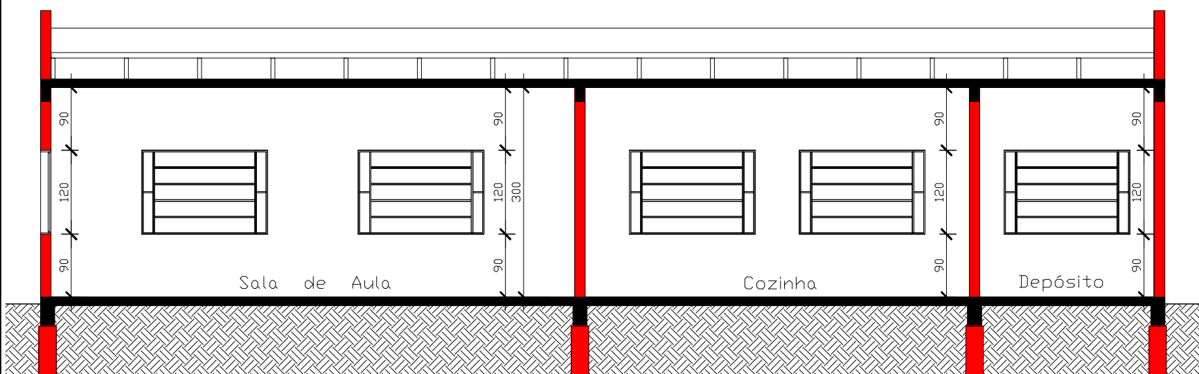
CORTE AA'
