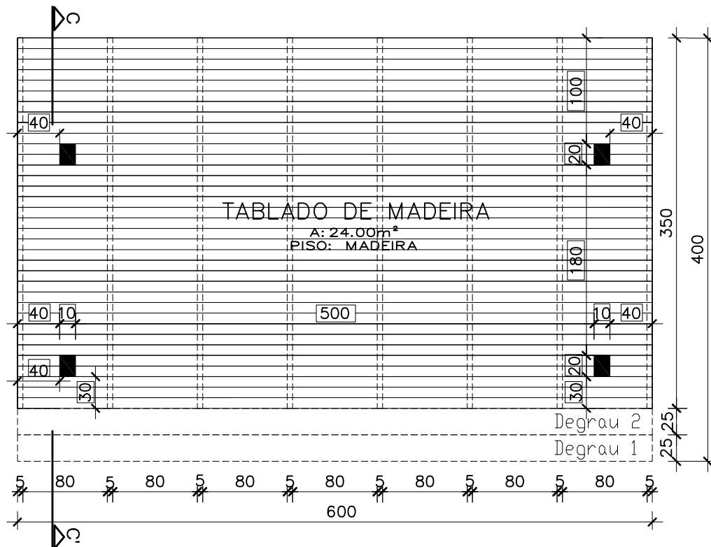
PLANTA BAIXA TABADO
