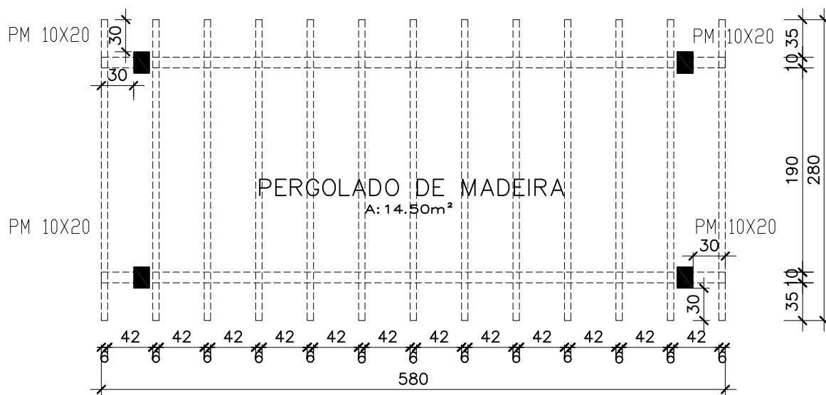
PLANTA BAIXA PERGOLADO
